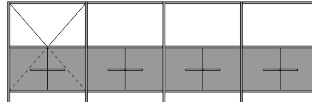
Композиция № 31 L 2788 mm B 360 mm H 917 mm
