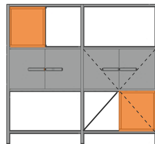
Композиция № 12 L 1404 mm B 360 mm H 1313 mm
