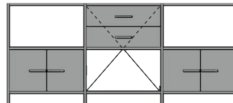
Композиция № 9 L 2096 mm B 360 mm H 917 mm
