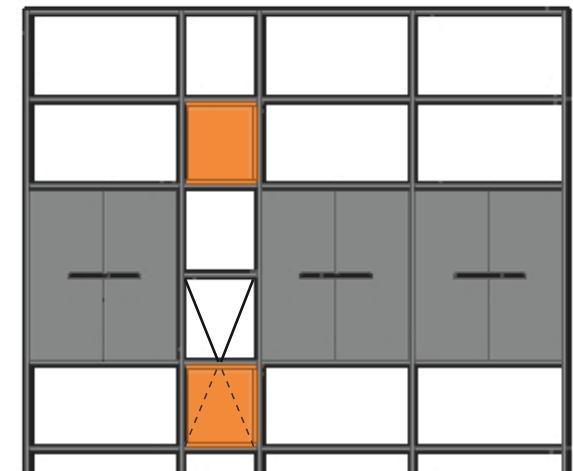
Композиция № 26 L 2452 mm B 360 mm H 2105 mm
